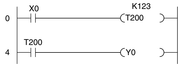
Релейная диаграмма
