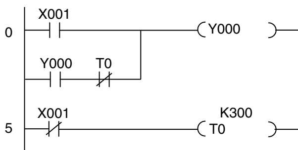
Релейная диаграмма
