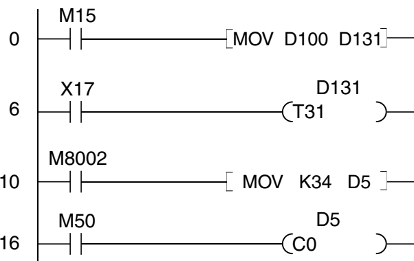
Релейная диаграмма
