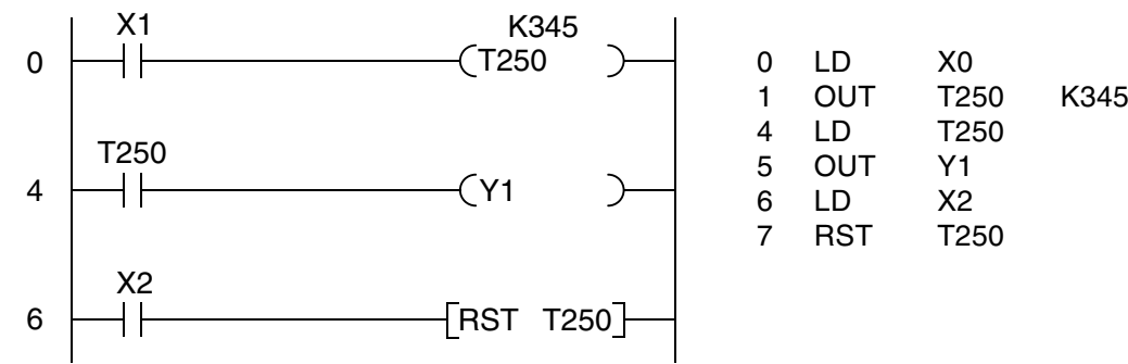
Релейная диаграмма
