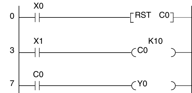
Релейная диаграмма
