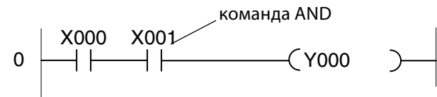
Релейная диаграмма
