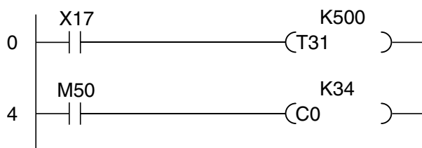
Релейная диаграмма
