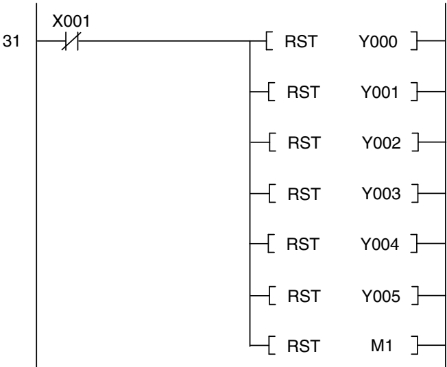
Релейная диаграмма
