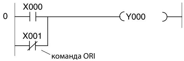
Релейная диаграмма
