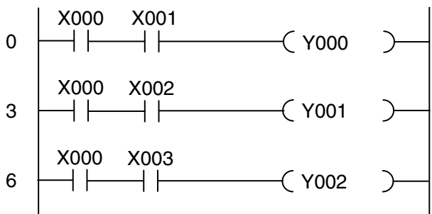
Релейная диаграмма
