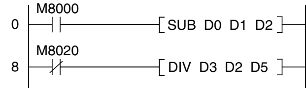
Релейная диаграмма
