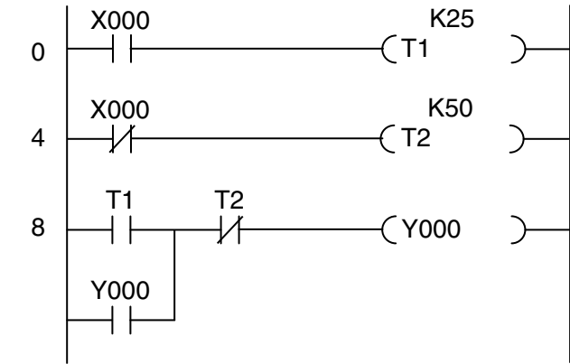
Релейная диаграмма
