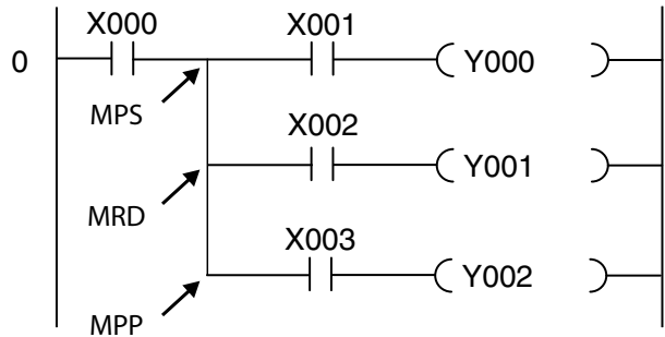
Релейная диаграмма
