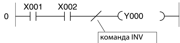
Релейная диаграмма
